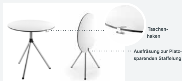
Mollinaro BIT | Klapp-Bistrotisch Tischplatte weiss | auf- und zugeklappter Zustand mit Ausfräsung
